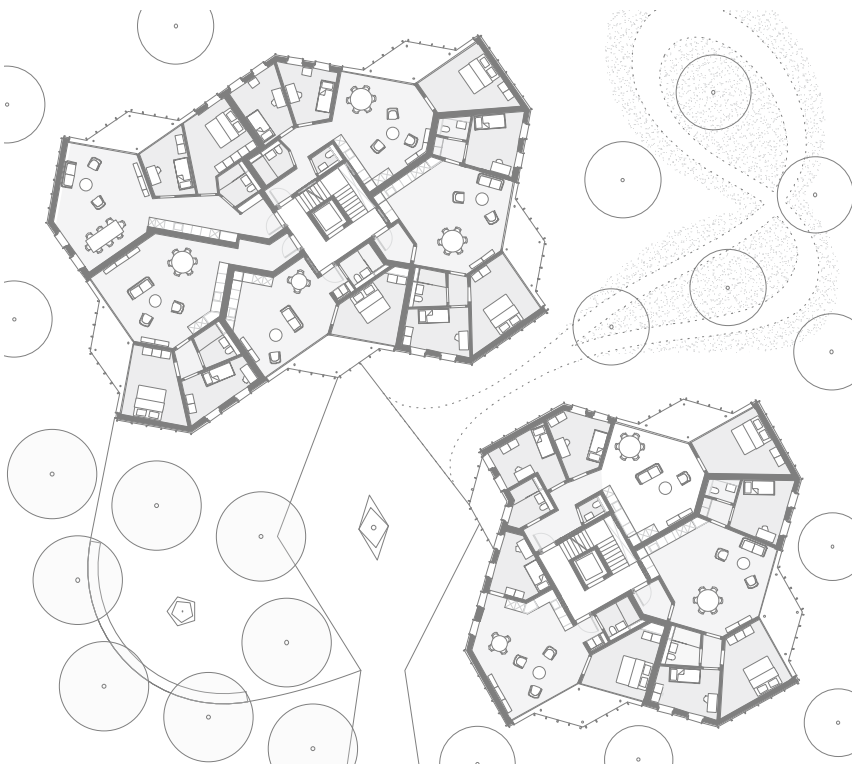
Regelgeschoss
